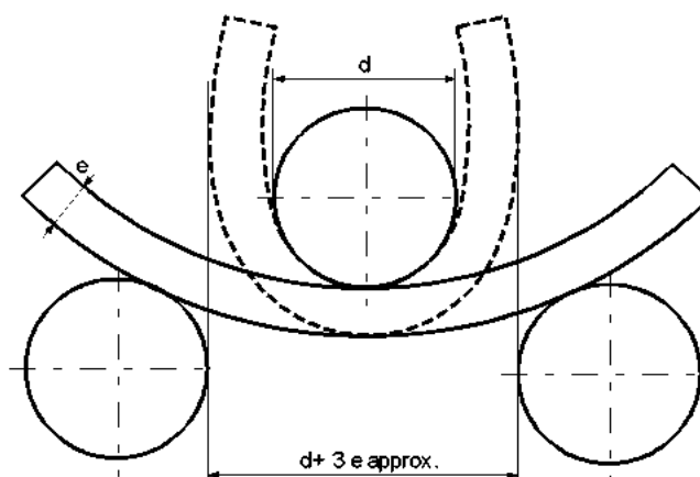
Diagram ispitivanja na savijanje
